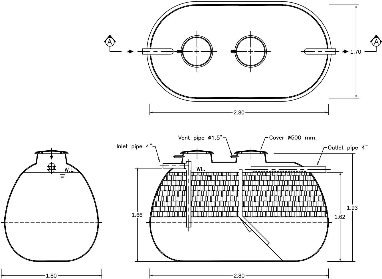
SECTION A-A
