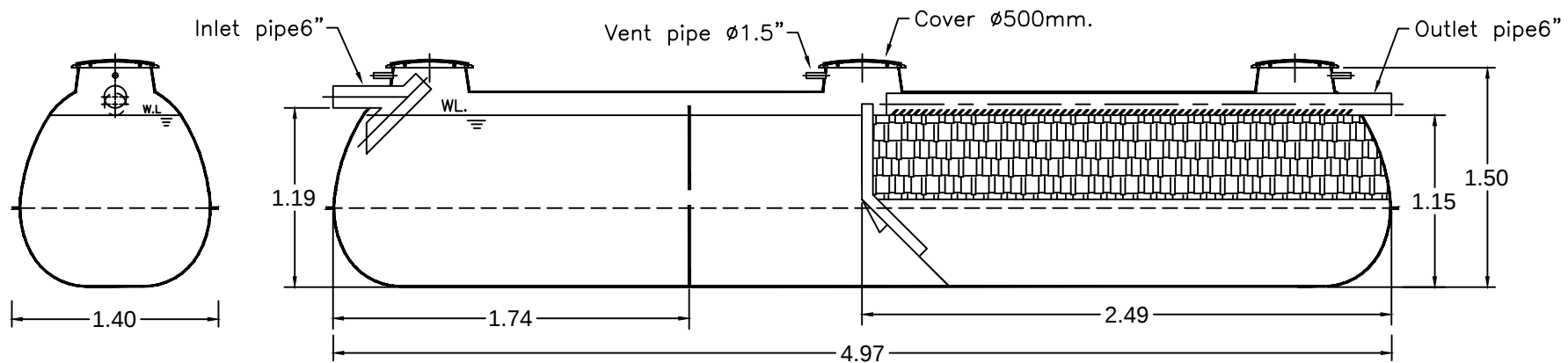
SECTION A-A
