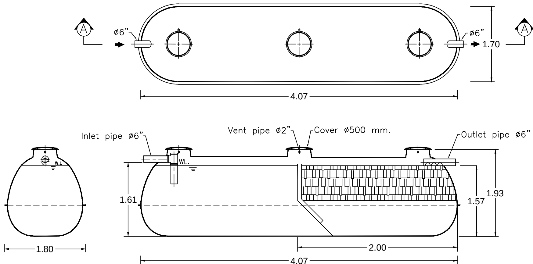
SECTION A-A
