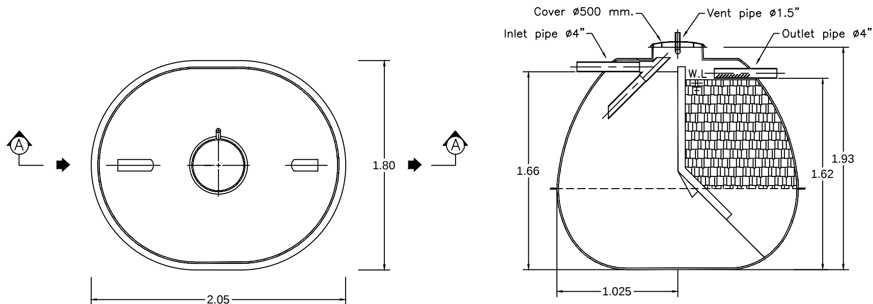
SECTION A-A
