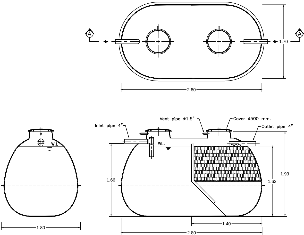
SECTION A-A
