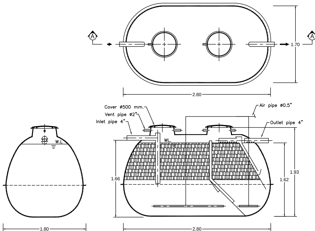
SECTION A-A
