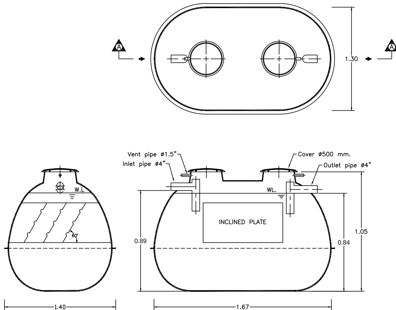
SECTION A-A
