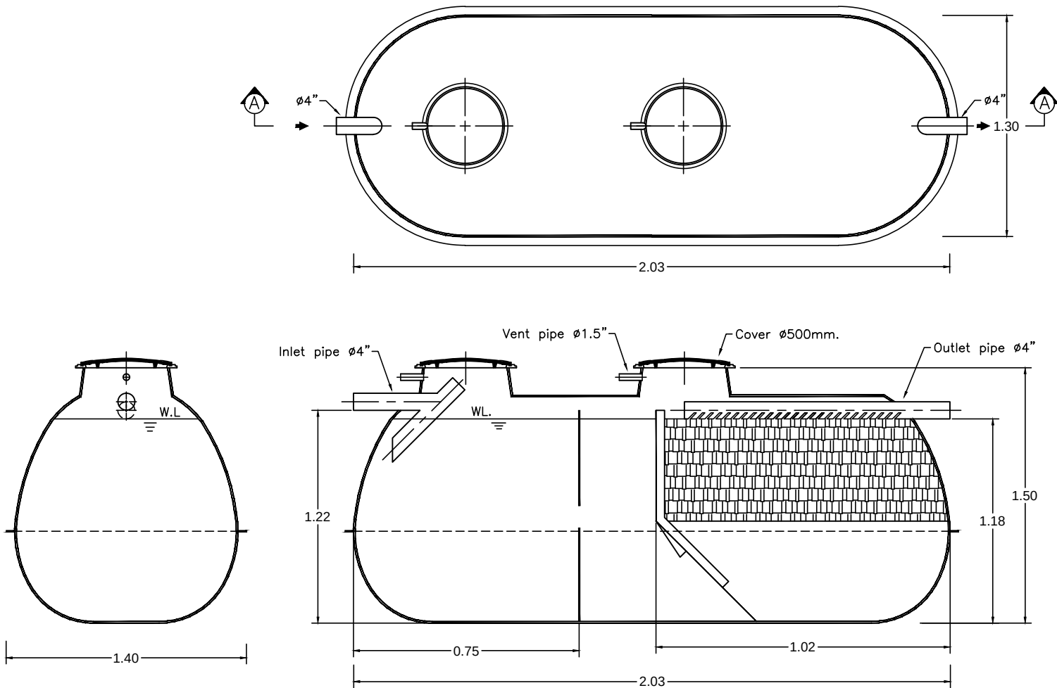
SECTION A-A
