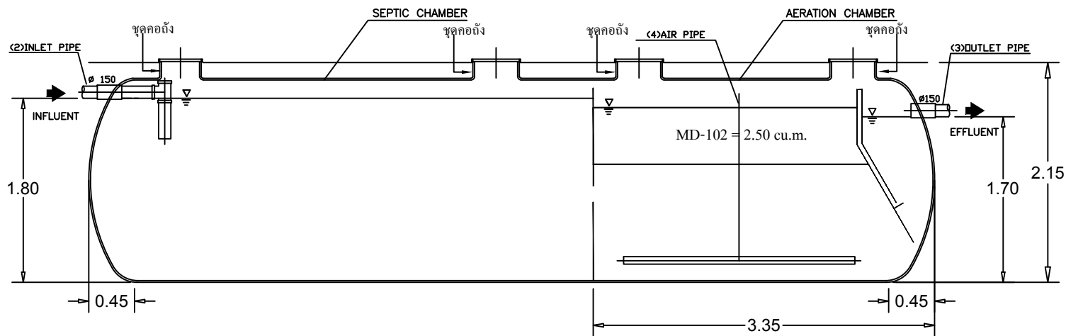
SECTION A-A
