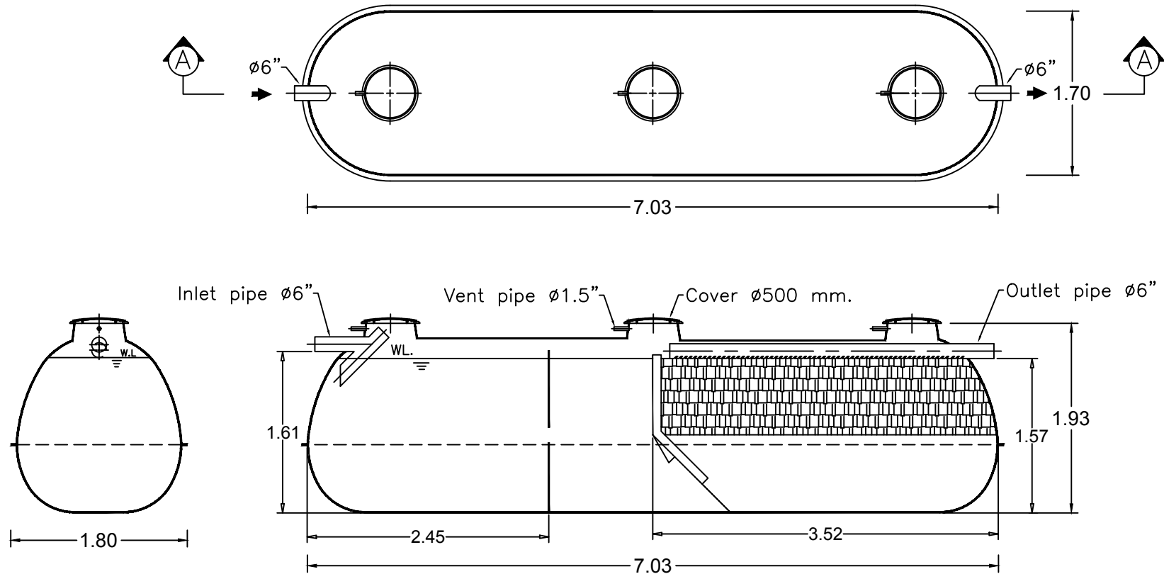
SECTION A-A
