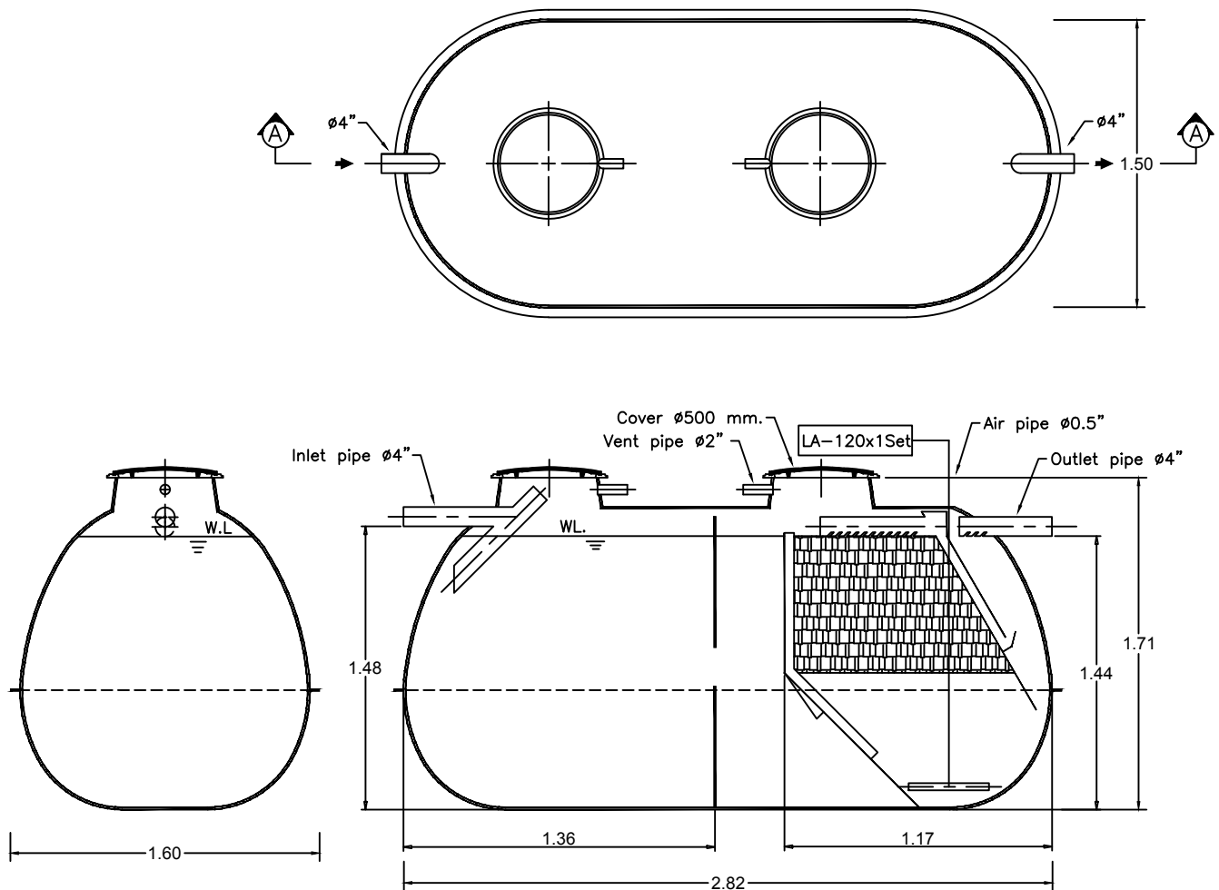
SECTION A-A
