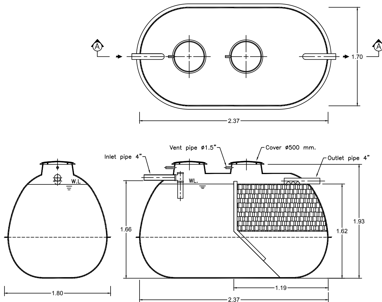
SECTION A-A
