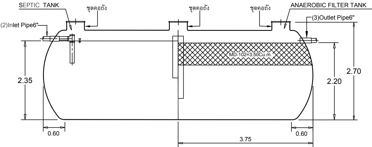
SECTION A-A
