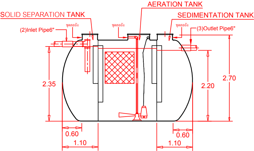
SECTION A-A
