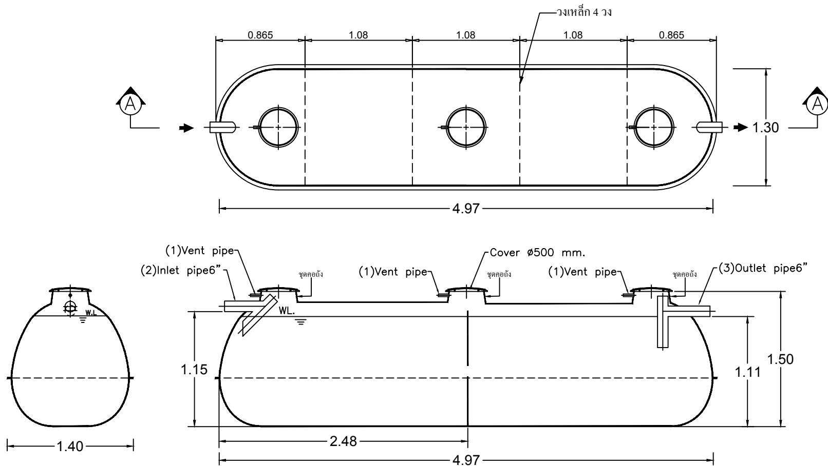
SECTION A-A
