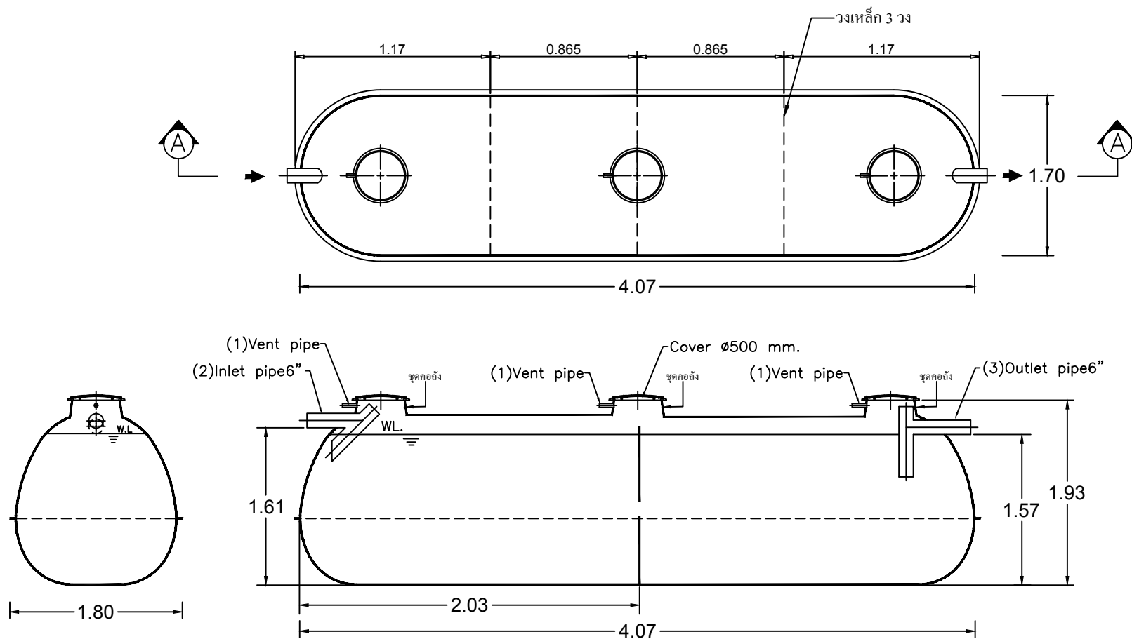
SECTION A-A
