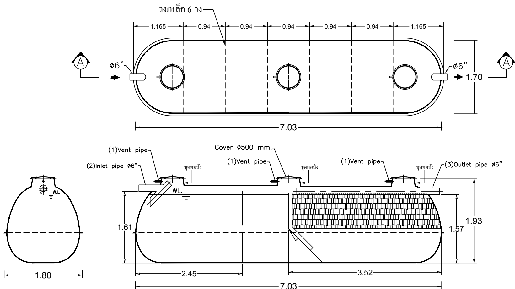
SECTION A-A
