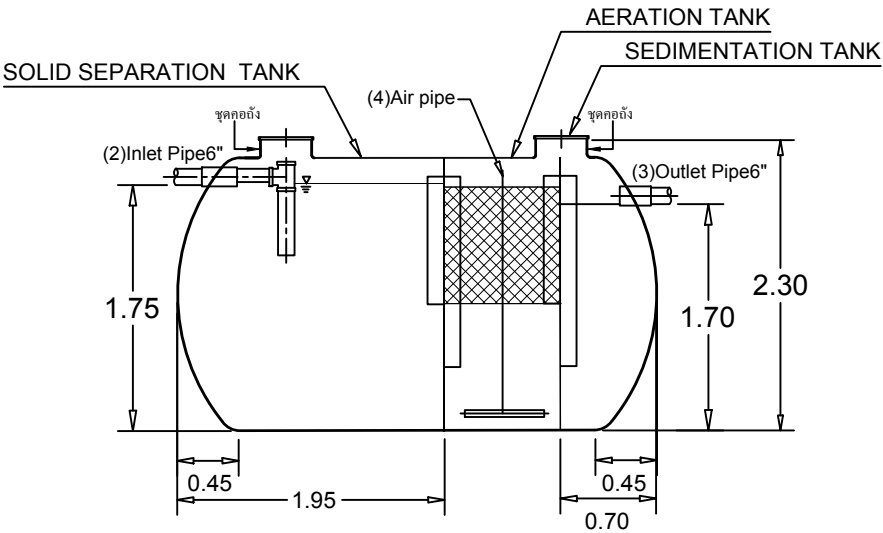
SECTION A-A
