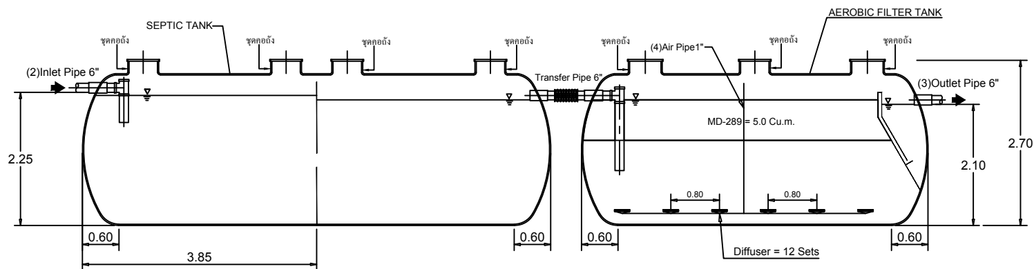
SECTION A-A
