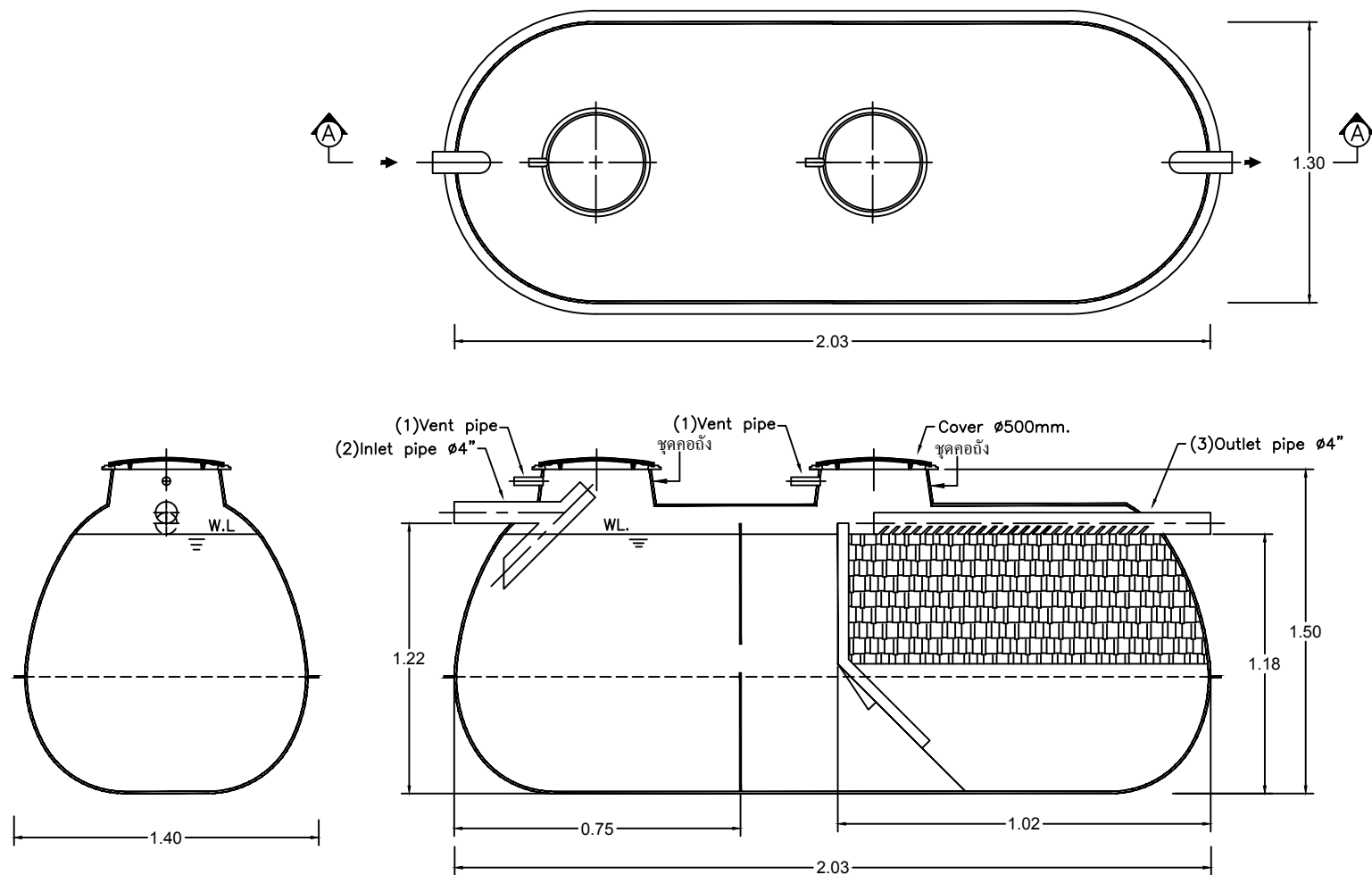
SECTION A-A
