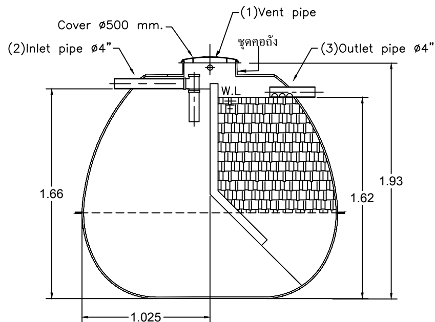
SECTION A-A
