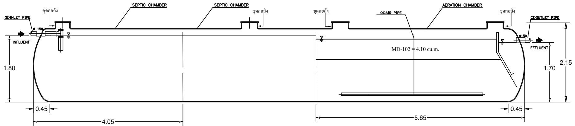
SECTION A-A
