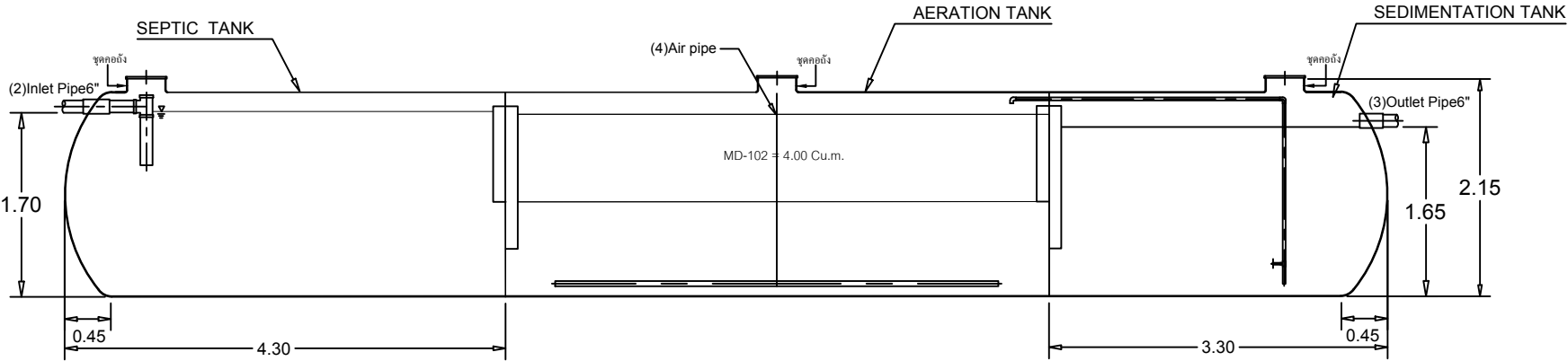
SECTION A-A
