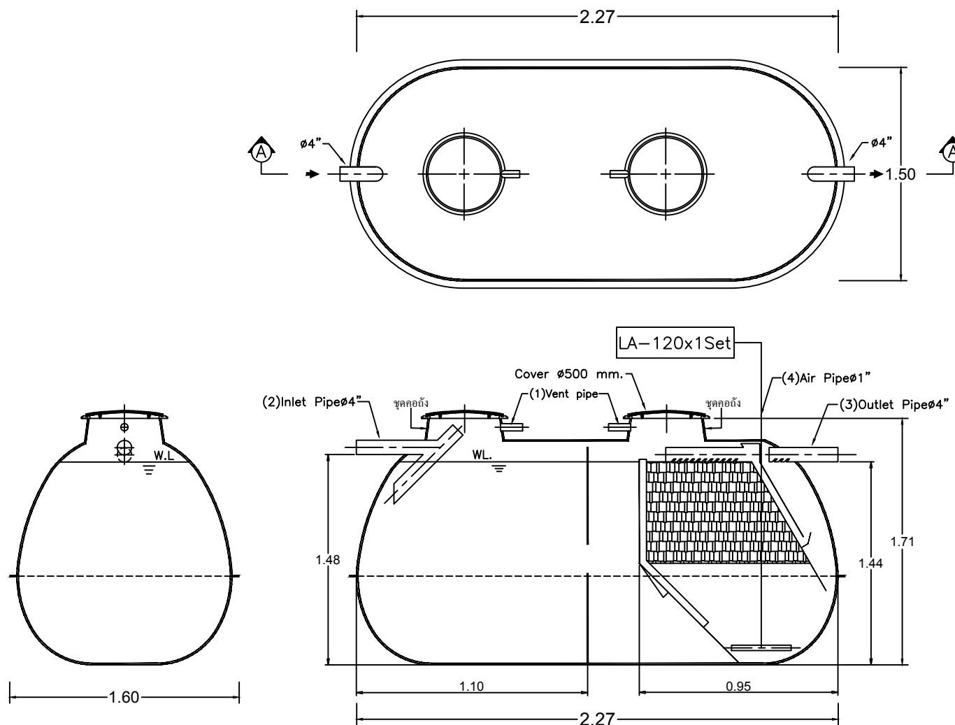
SECTION A-A
