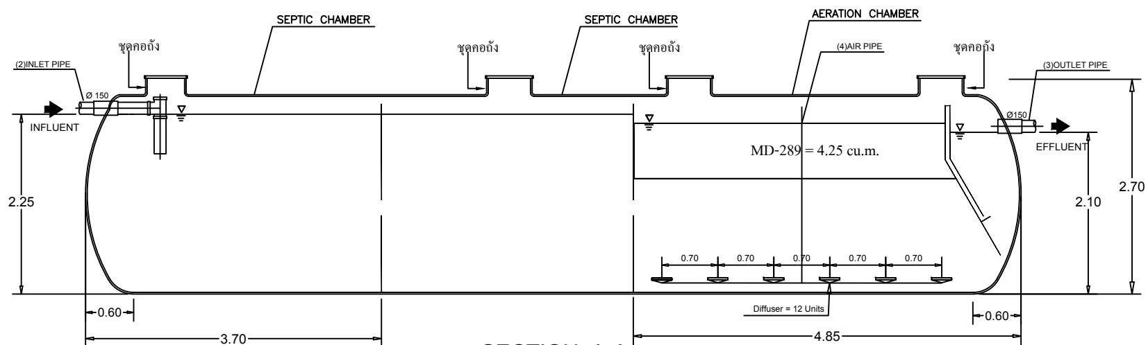
SECTION A-A
