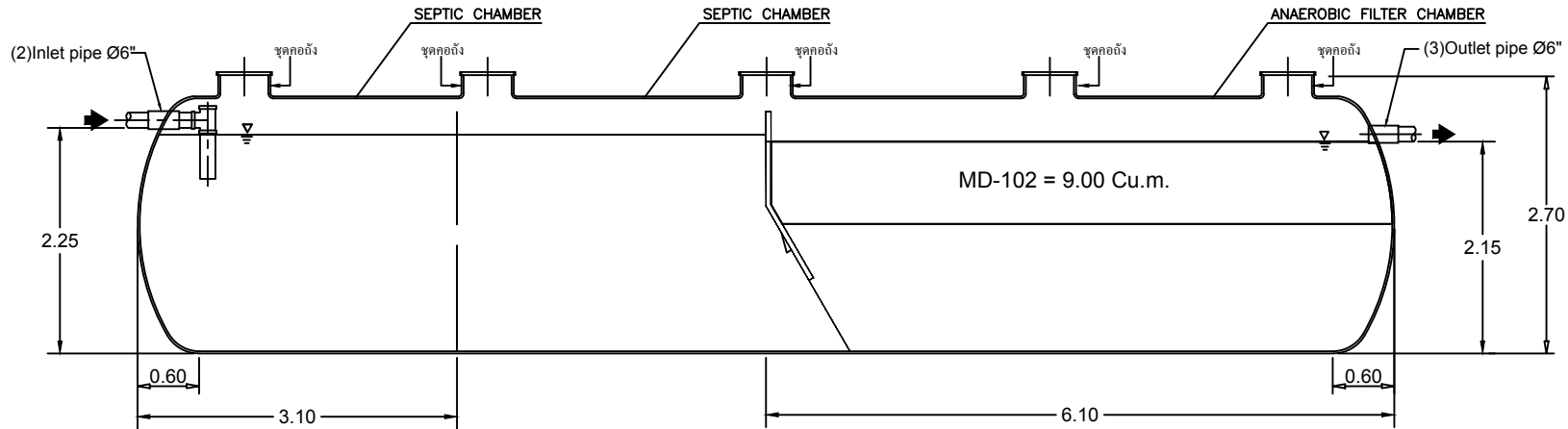
SECTION A-A
