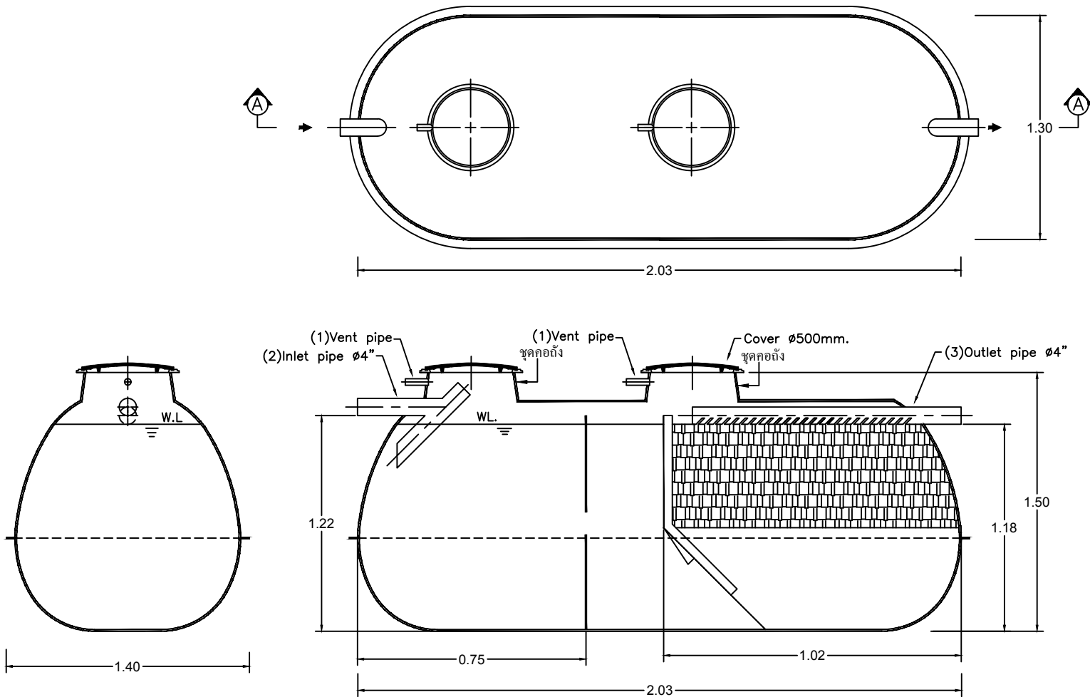
SECTION A-A
