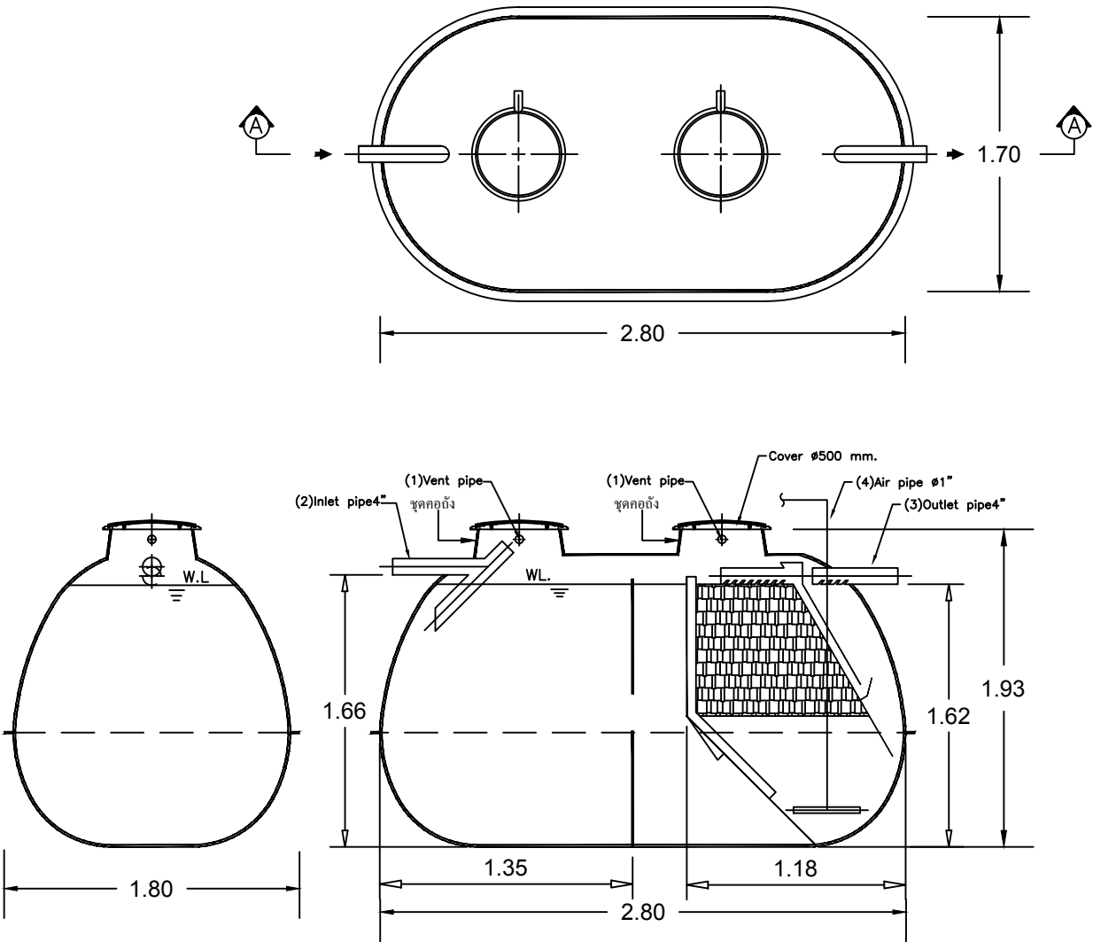
SECTION A-A
