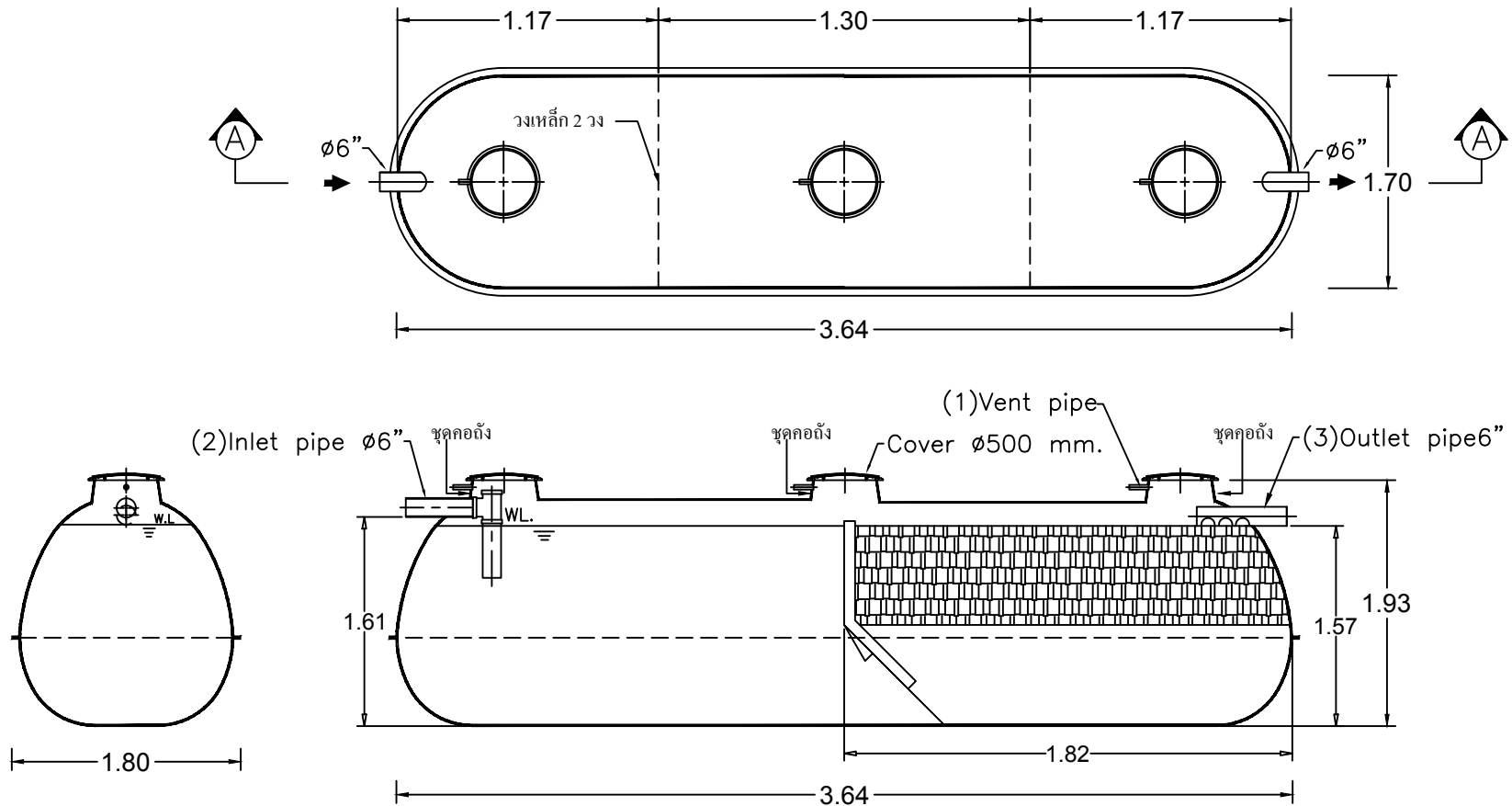
SECTION A-A
