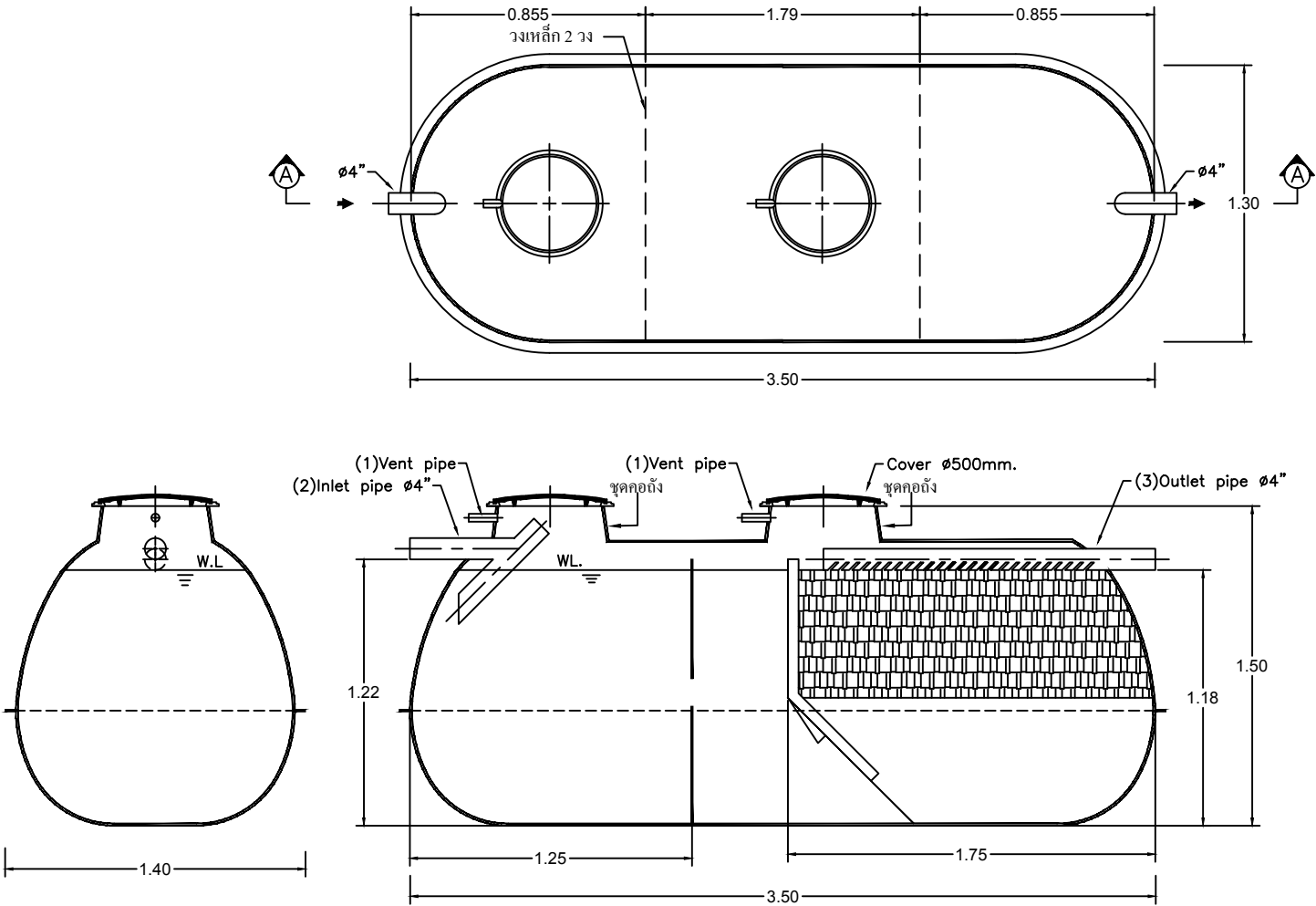
SECTION A-A
