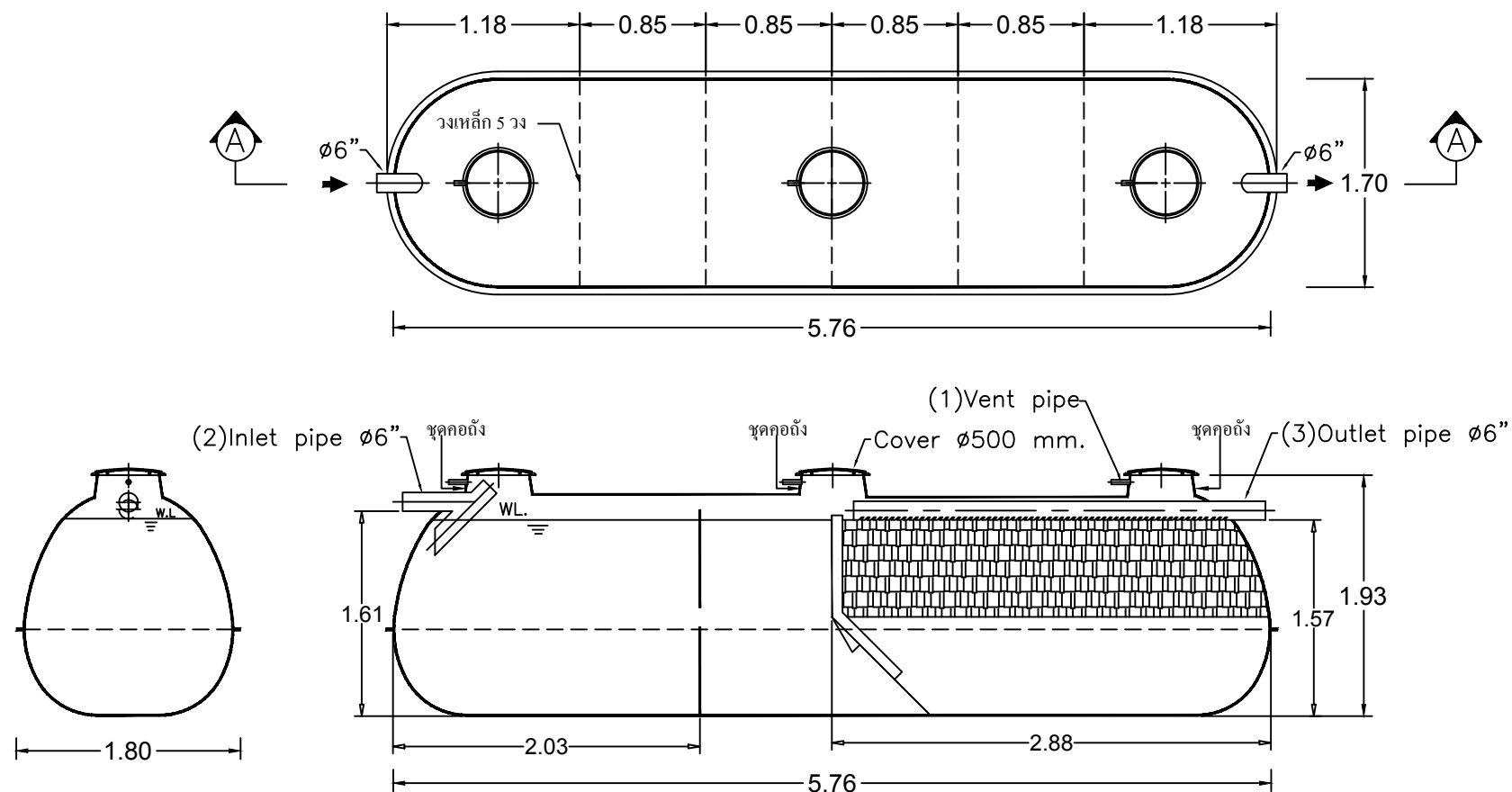
SECTION A-A
