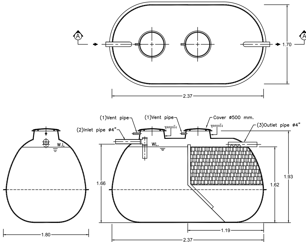
SECTION A-A
