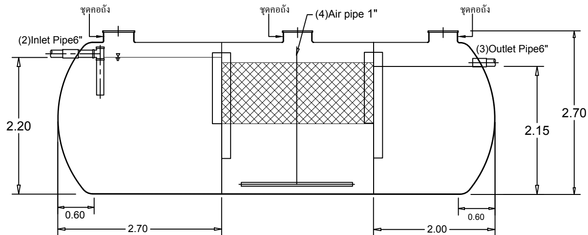
SECTION A-A
