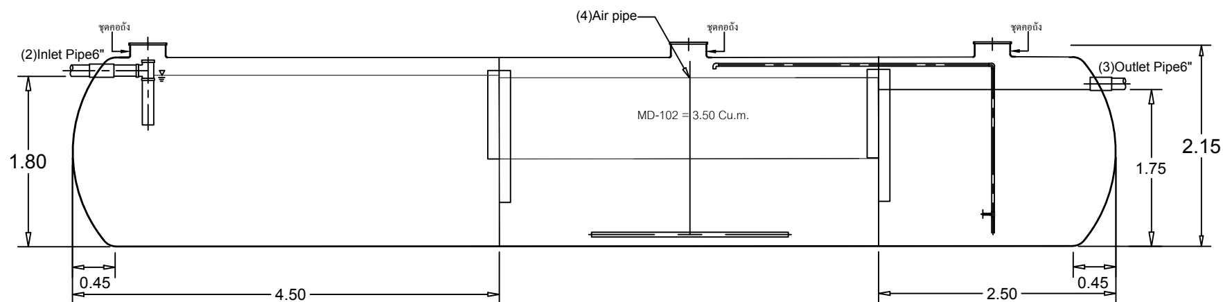
SECTION A-A
