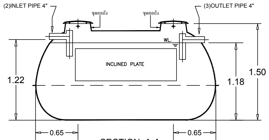
SECTION A-A
