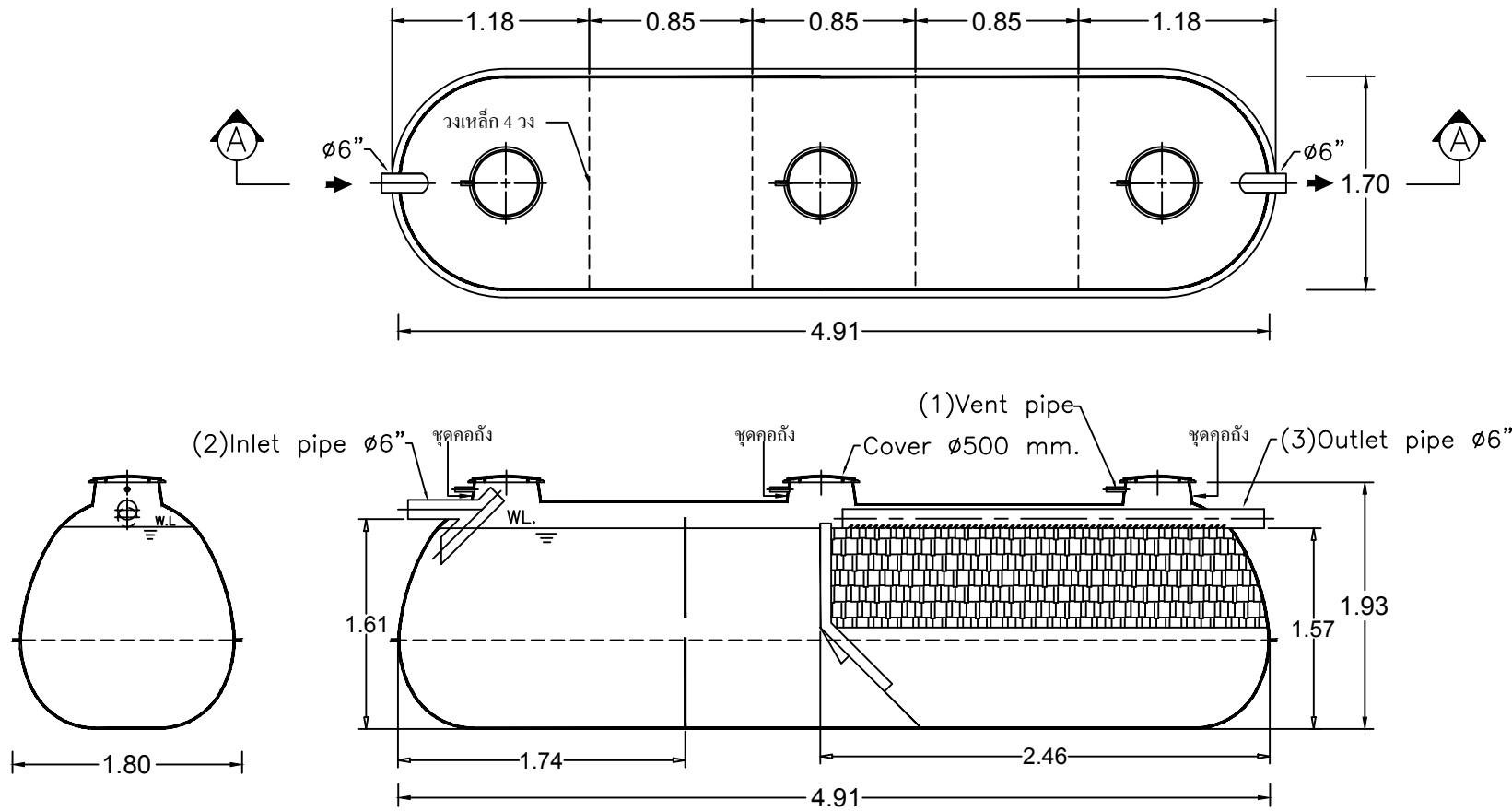
SECTION A-A
