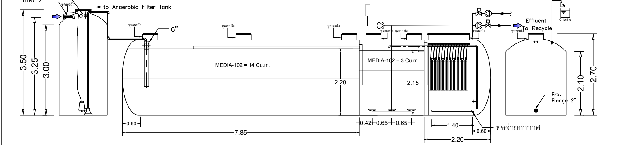
SECTION A-A
