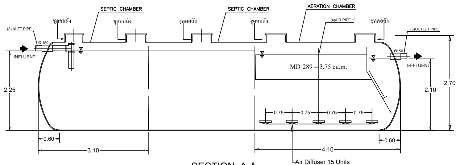
SECTION A-A
