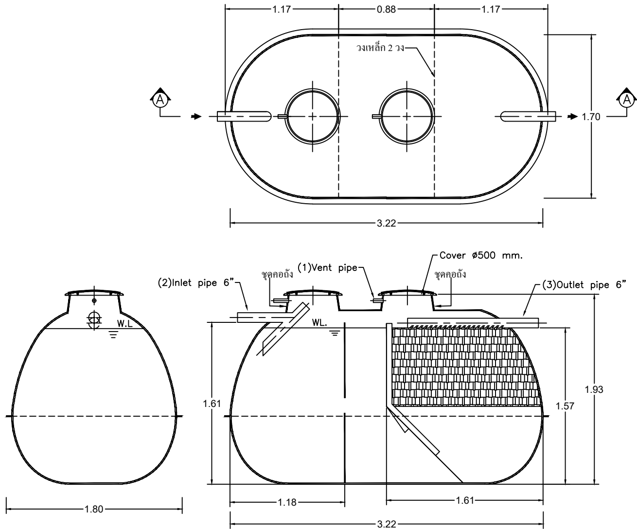
SECTION A-A
