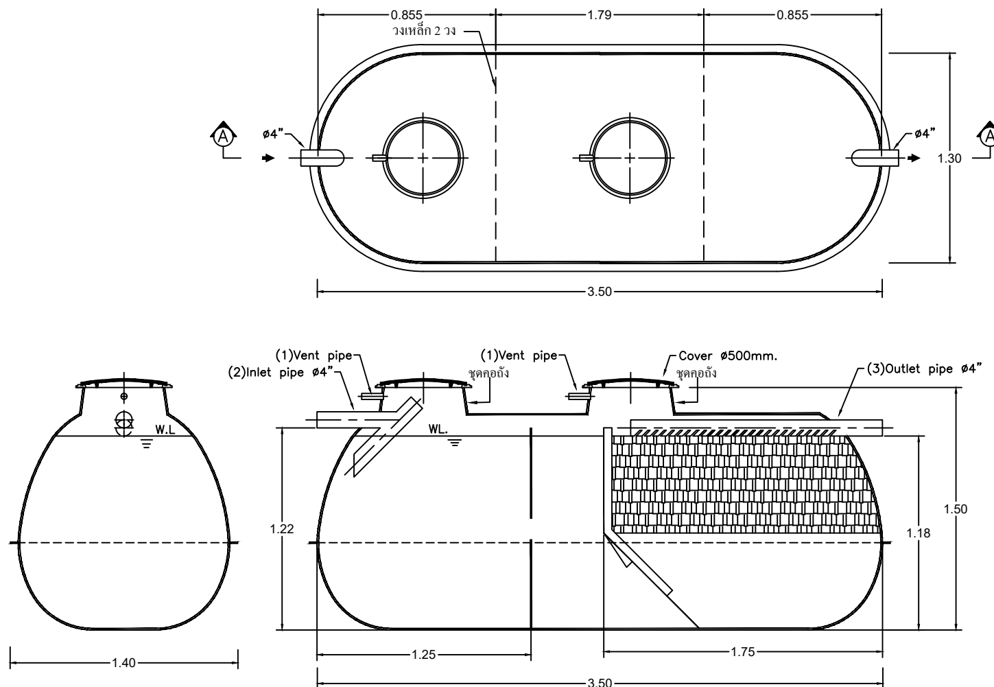
SECTION A-A
