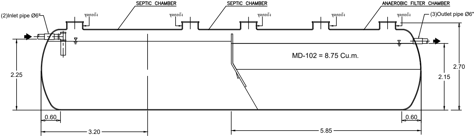
SECTION A-A
