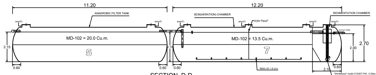
SECTION D-D
