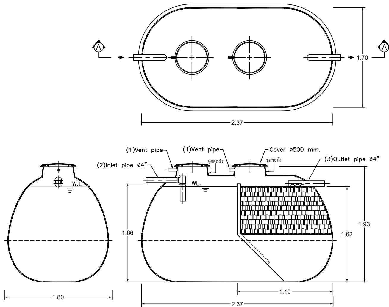
SECTION A-A
