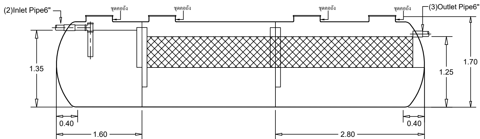
SECTION A-A
