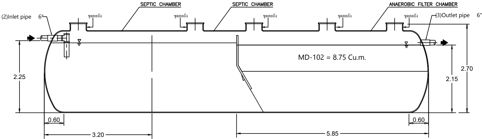
SECTION A-A
