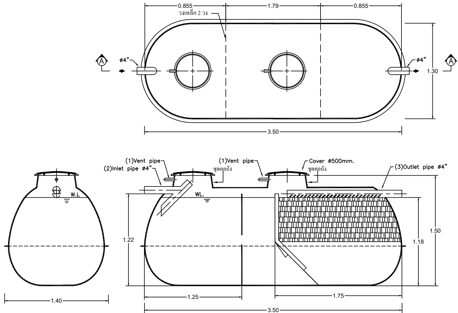
SECTION A-A
