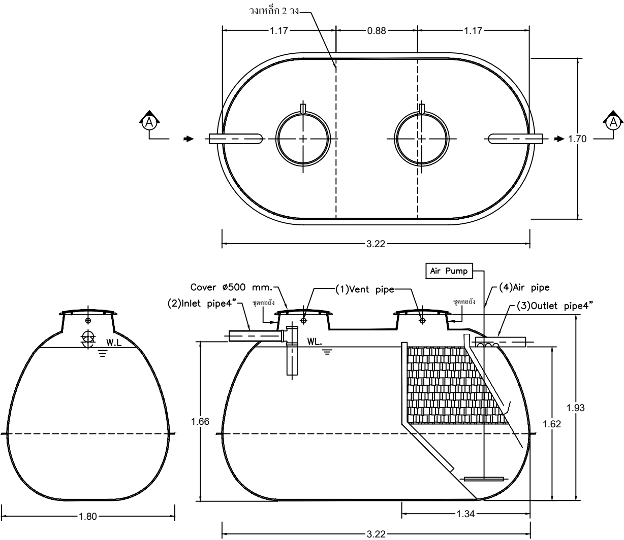
SECTION A-A
