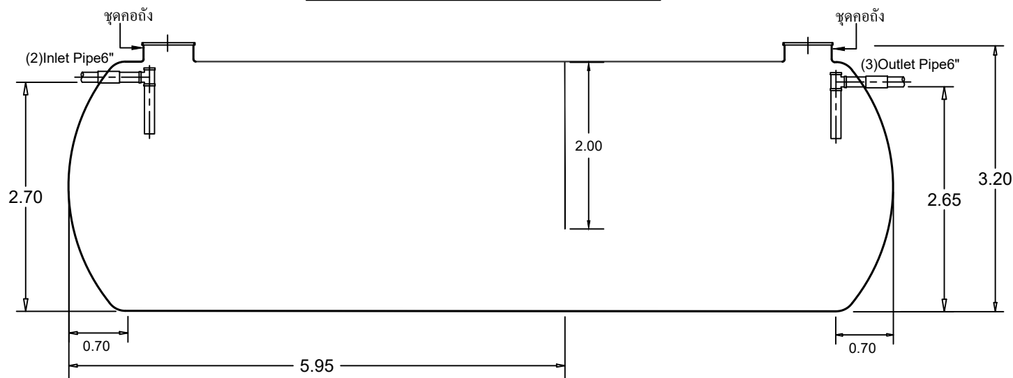
SECTION A-A
