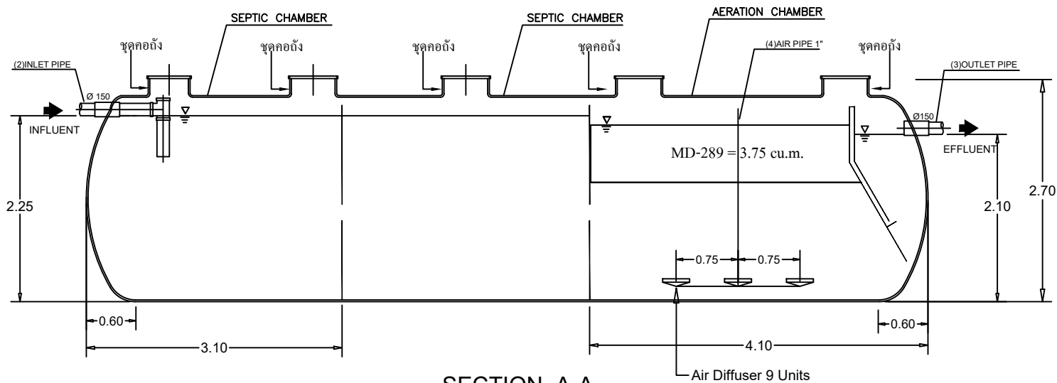
SECTION A-A
