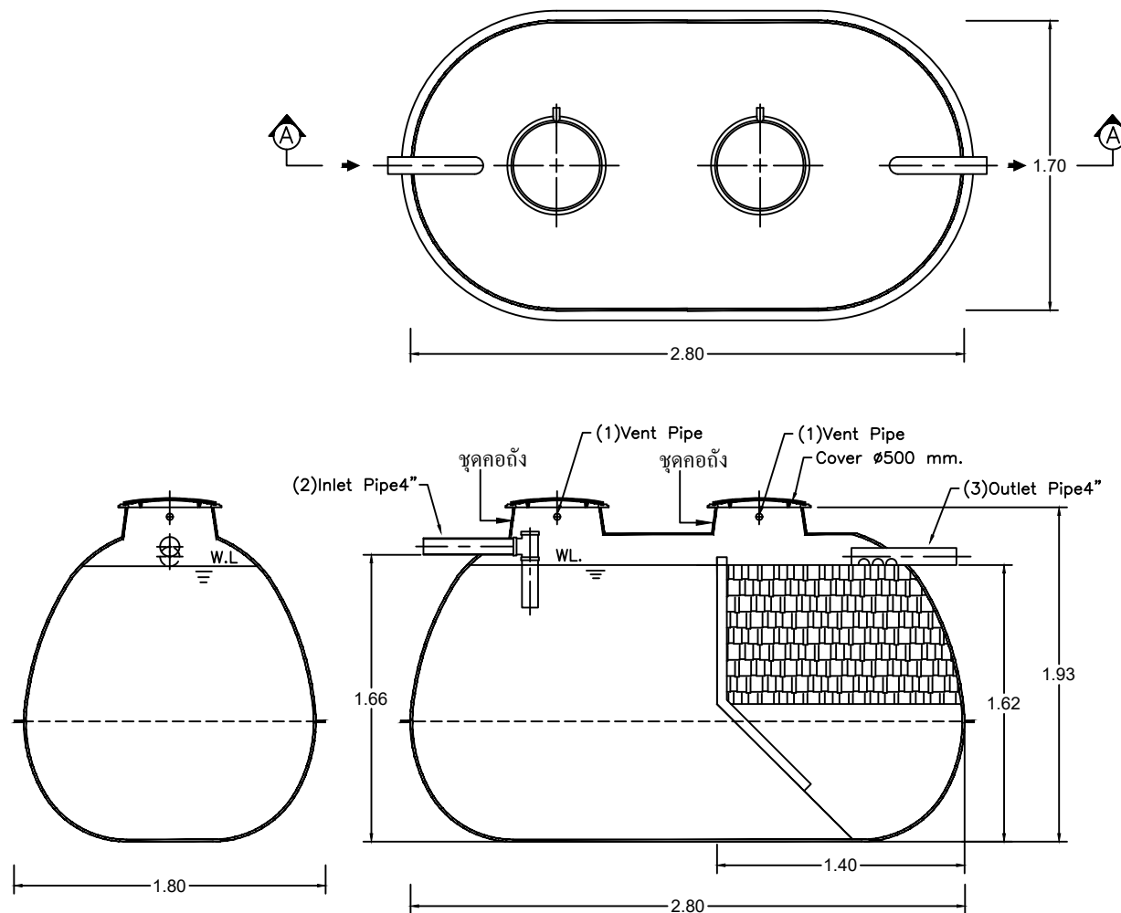
SECTION A-A
